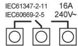
Anschlussplan RM16 HS WE
