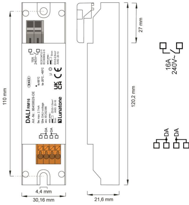
Geometrie RM16 DE
