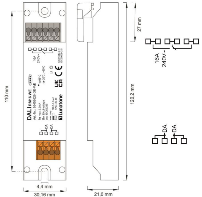
Geometrie RM16 DE WE
